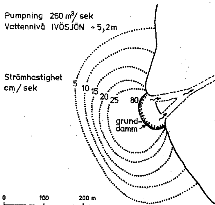
Fig. 14 Strömhastigheter vid pumpning - alternativ C (efter Larsson m.fl. 1976).
